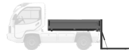
LP - Ladebordwand an Pritsche
